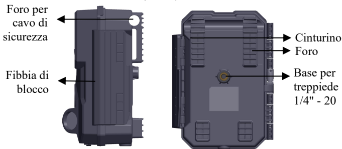
Figura 3: Vista destra/posteriore
