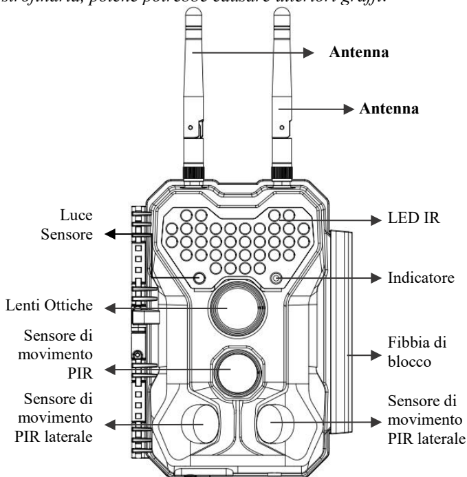
Figura 1: Vista frontale
