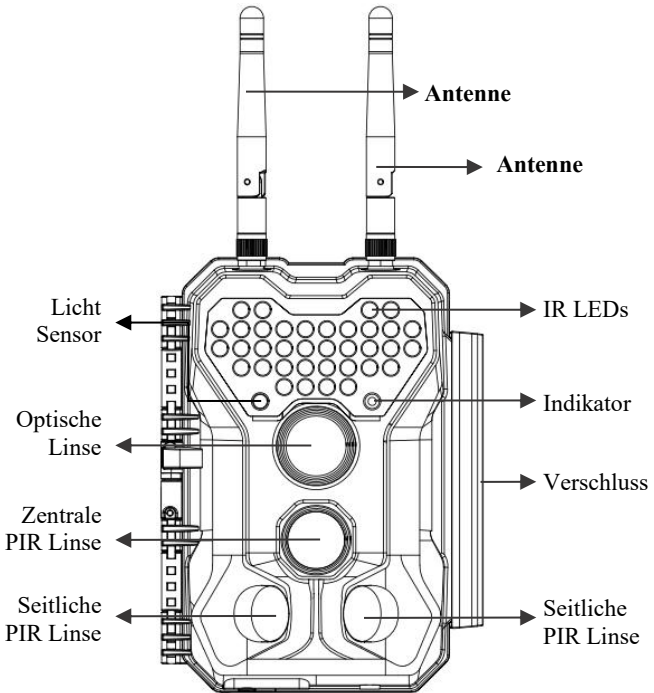
Abb. 1: Vorderansicht
