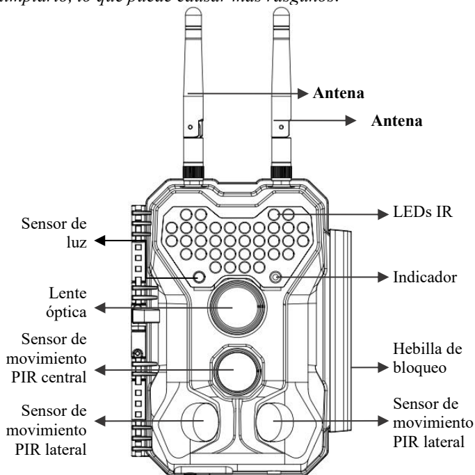
Figura 1: Vista frontal
