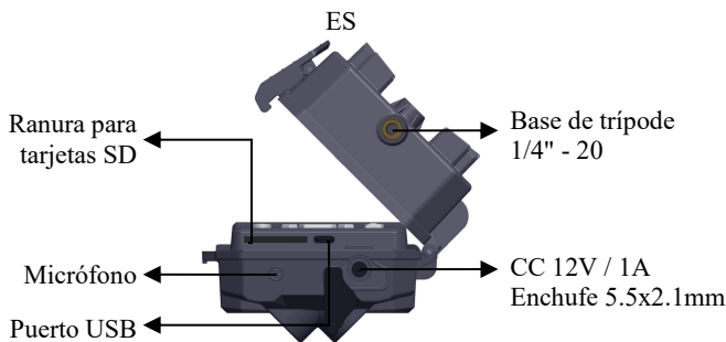
Figura 2: Vista inferior
